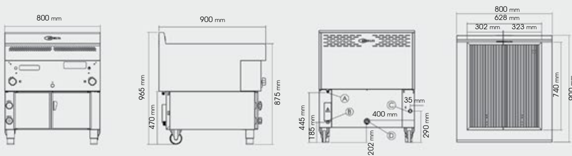
GHPI 2/800
